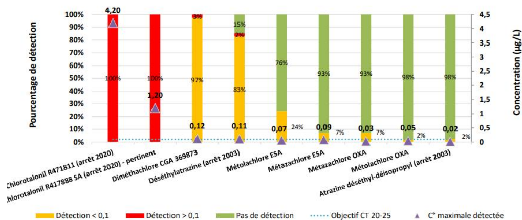
Détection des molécules récurrentes au droit du captage F3 Lutineaux Période 2020-2025
